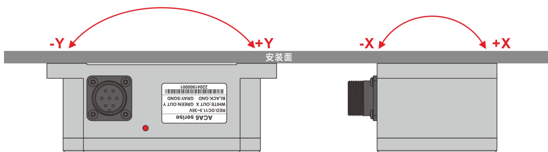
水平向下安装
