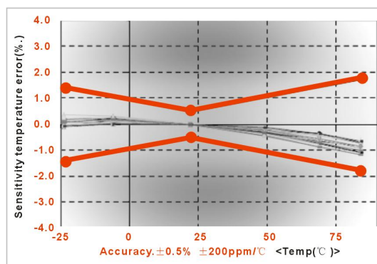
2: 温度特性图:
