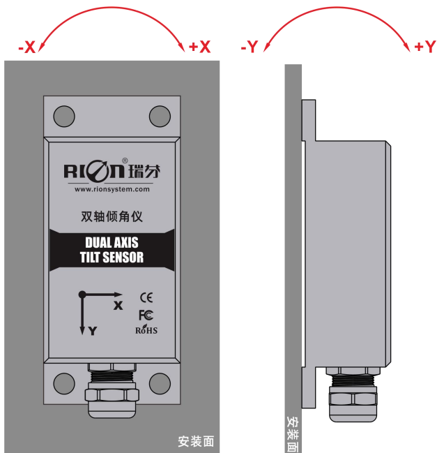
垂直安装
