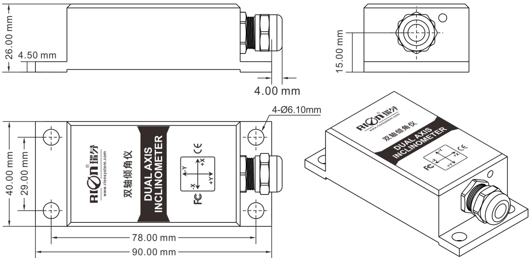
外壳封装尺寸图
